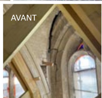
Consolidation des clés de voûtes par l'injection de chaux qui a permis de remonter la structure affaïssée
